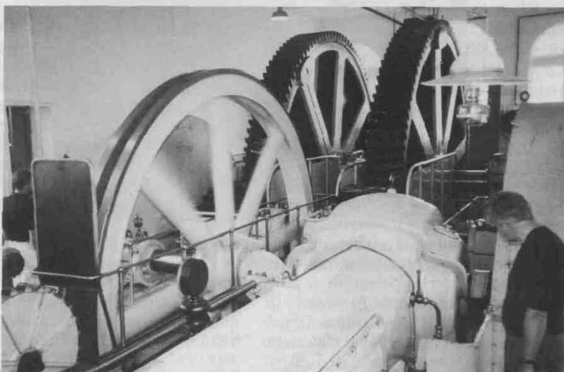
De gigantische landraders en het grote vlieg wiel van het stoomgemaal Halfweg, daterende uit 1888. Bezigting is zeer de moeite waard. Het geniaal is periodiek in gebruik t.h.v. geïnteresseerden (opname: aug.1992).
